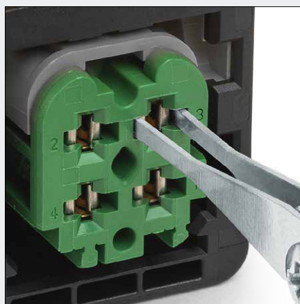
Вставка подходящего инструмента и расфиксация контакта
