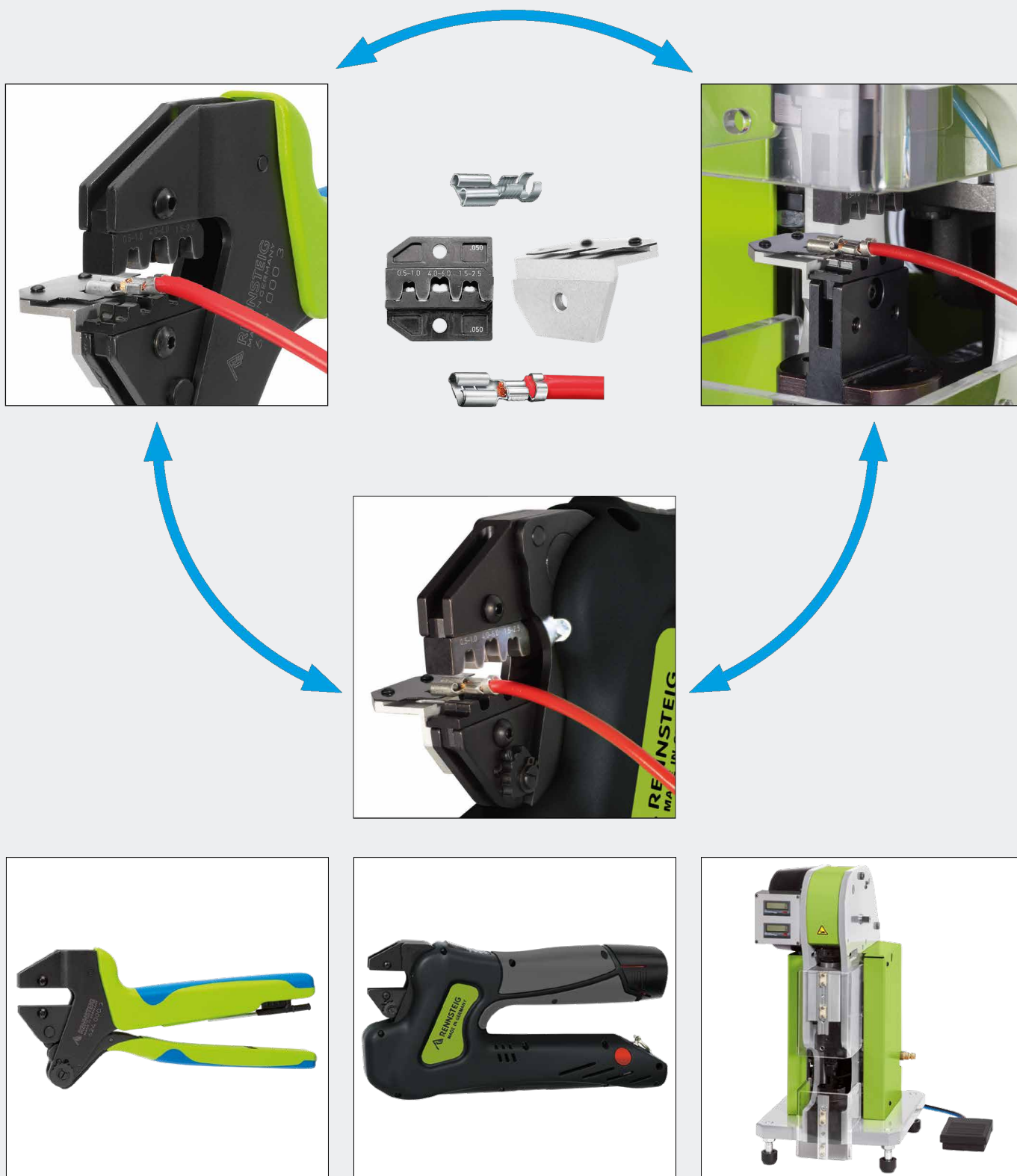
Многосистемные пресс-клещи PEW 12
