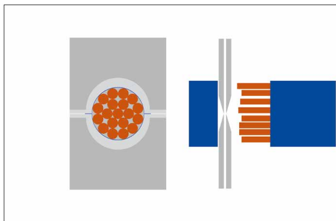
Снятие изоляции с помощью фасонных ножей
