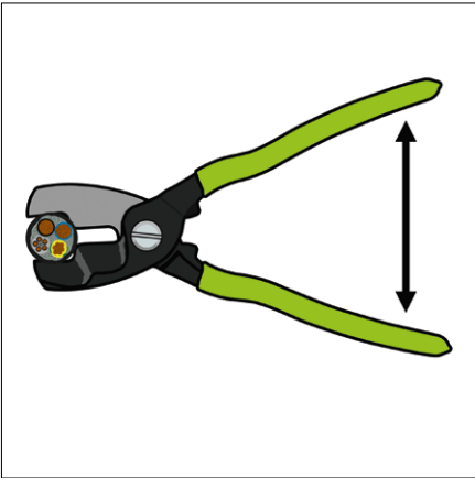
Этап 1: Предварительный рез. За счет использования передней режущей кромки удобная ширина рукоятки сохраняется при работе с кабелем большого диаметра
