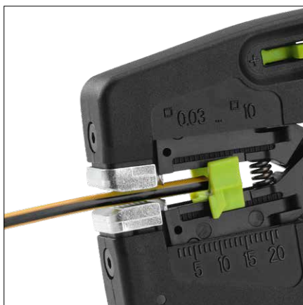
Металлические зажимные губки и легко регулируемый ограничитель длины для автоматического снятия изоляции
