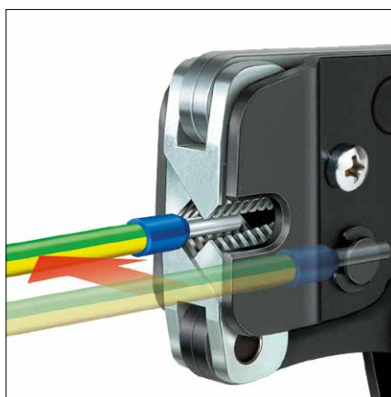
Номер арт. 610 087 3 боковая установка макс. до 2,5 мм 2
