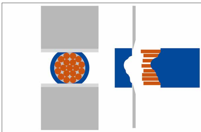
Снятие изоляции с автоматической настройкой
