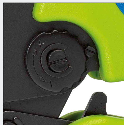
Принудительное завершение процесса обжима (с аварийной разблокировкой), регулируемое давление обжима
