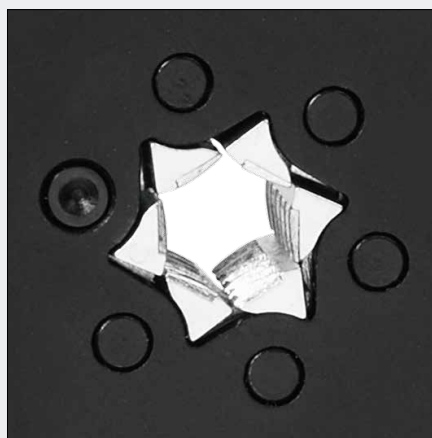
Шестигранная форма обжима – автоматическая настройка макс. до 16 мм 2 / AWG 6
