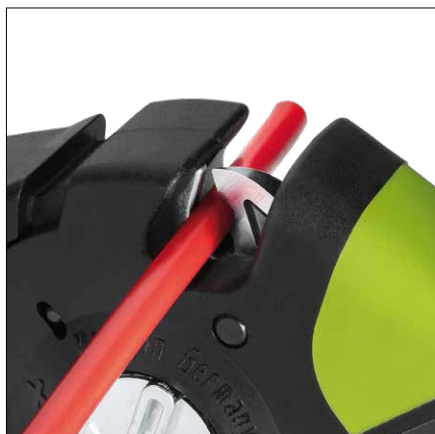
Отрезание кабеля
